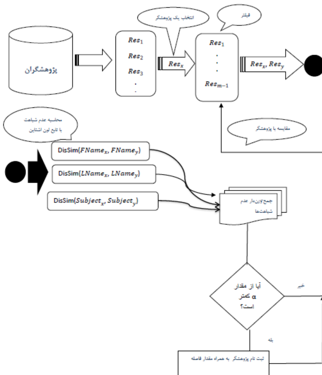
شکل ۸- فلوچارت چارچوب استفاده شده
